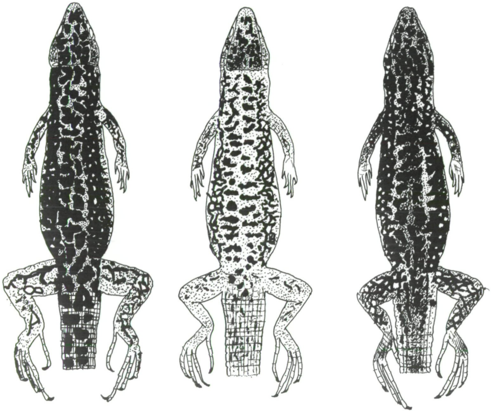
Fig. 5: Pattern variability in ' Lacerta ' cyreni castiliana ssp. nov. from Gredos, I. Abb. 5: Zeichnungsvariabilität bei ' Lacerta ' cyreni castiliana ssp. nov. von Gredos, I.
